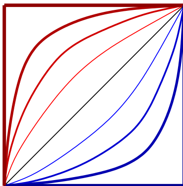
Homotopie \mathcal{F} -continue passant de \lfloor à \lrcorner
