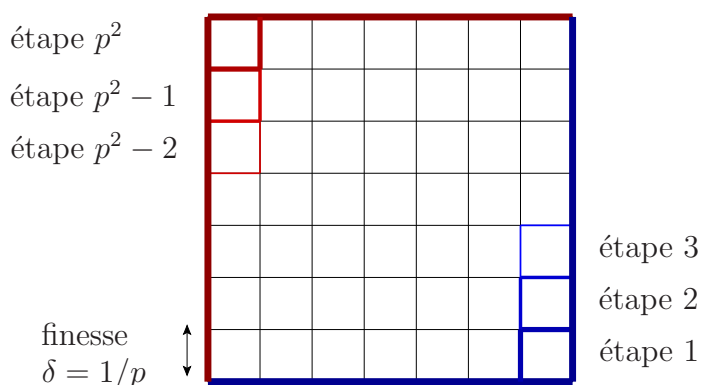
(1, \mathbf{M}) -homotopie passant de \lfloor à \lrcorner pour la finesse \delta
